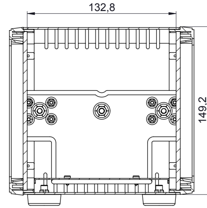
KESIT A-A
