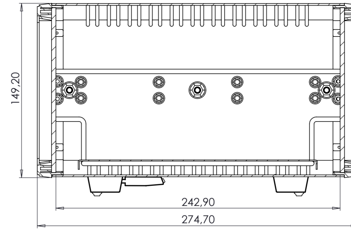
KESIT A-A
