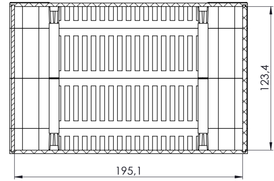
KESIT B-B
