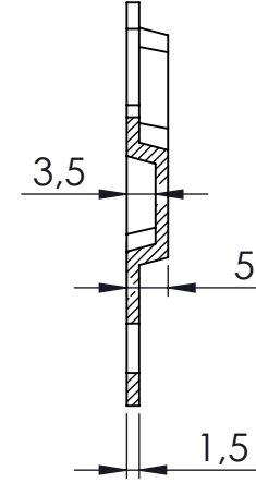
KESİT A-A
