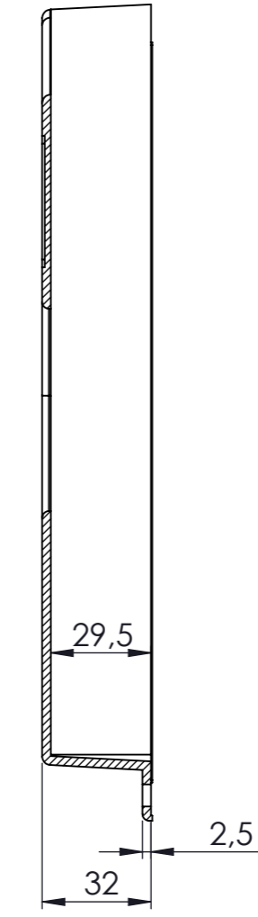
KESİT A-A
